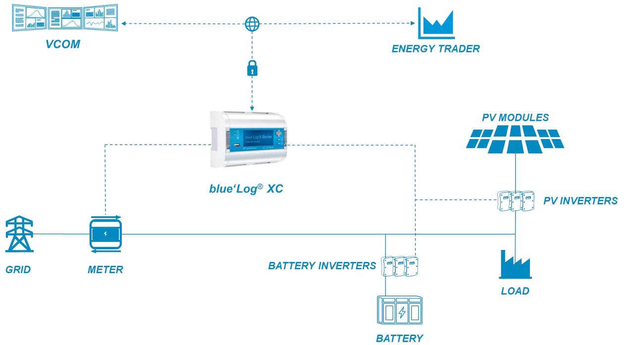
Beispiel für den Aufbau einer Anlage mit HEMS
